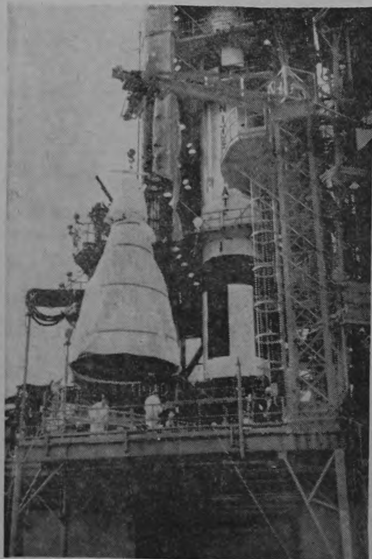
INSTALACION DE LA NAVE ESPACIAL. — En la fotografía se ve el vehículo espacial Géminis 9 en los momentos que es colocado sobre el cohete (que se ve parcialmente al fondo) en Cabo Kennedy, Florida. Desde esta instalación, la Cancha 19, el Géminis 9 comenzará su viaje de tres días por el espacio.
